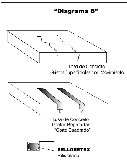
Diagramas relacionados a Especificación Técnica de Cisternas
